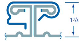
T-25b Flanged
