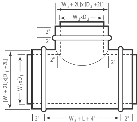
Tee
