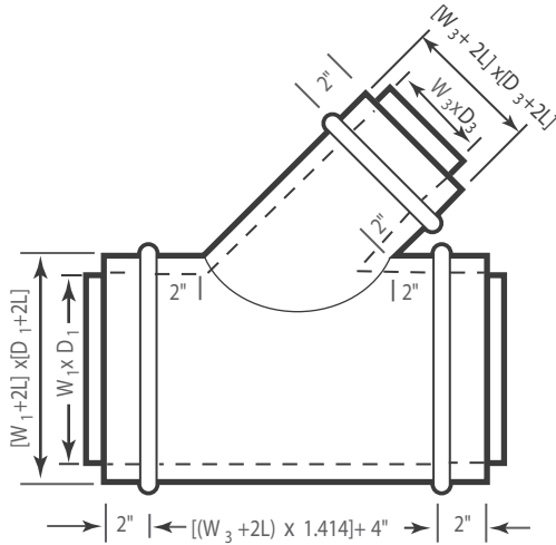
Lateral 45°
