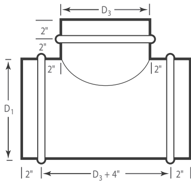
Tee
