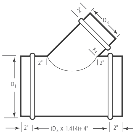
Lateral 45°
